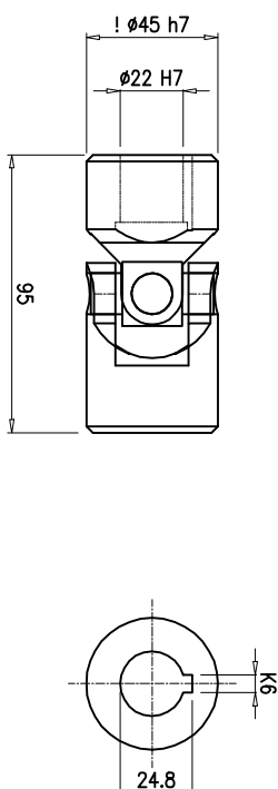
DIN 808-45-K22-95-EG QTY : 2 PCS
